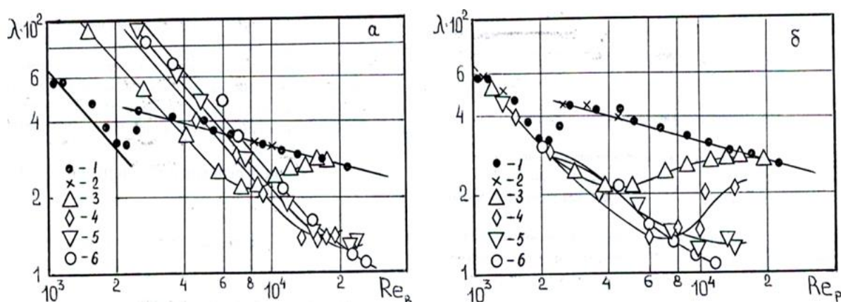
Рис. 3. Зависимость \lambda от Re : 1- вода; 2-6 – концентрация диталана OTS - C = 0,3; 0,6; 1,2; 1,8 и 2,4\% , вес., соответственно; концентрация хлористого натрия C = 3\% , вес.; температура раствора T = 18^\circ\text{C} . Числа Рейнольдса рассчитаны по вязкости воды (а) и раствора диталана OTS (б) соответственно. Данные работы [22]
