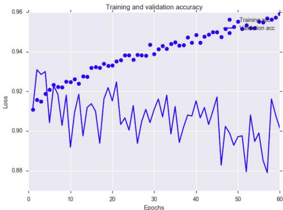
Рис. 3 Показатели работы многослойного перцептрона
