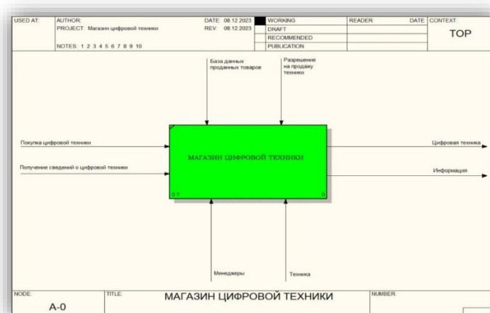
Рисунок 1 – Диаграмма нулевого уровня по методологии IDF0
