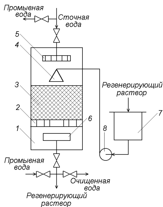
Рисунок 3.1 – Схема лабораторной установки для сорбционной очистки воды от нефтепродуктов: 1 – корпусная колонна; 2 – решетка; 3 – слой сорбента; 4,5,6 – распределители; 7 – бак с раствором; 8 – насос
